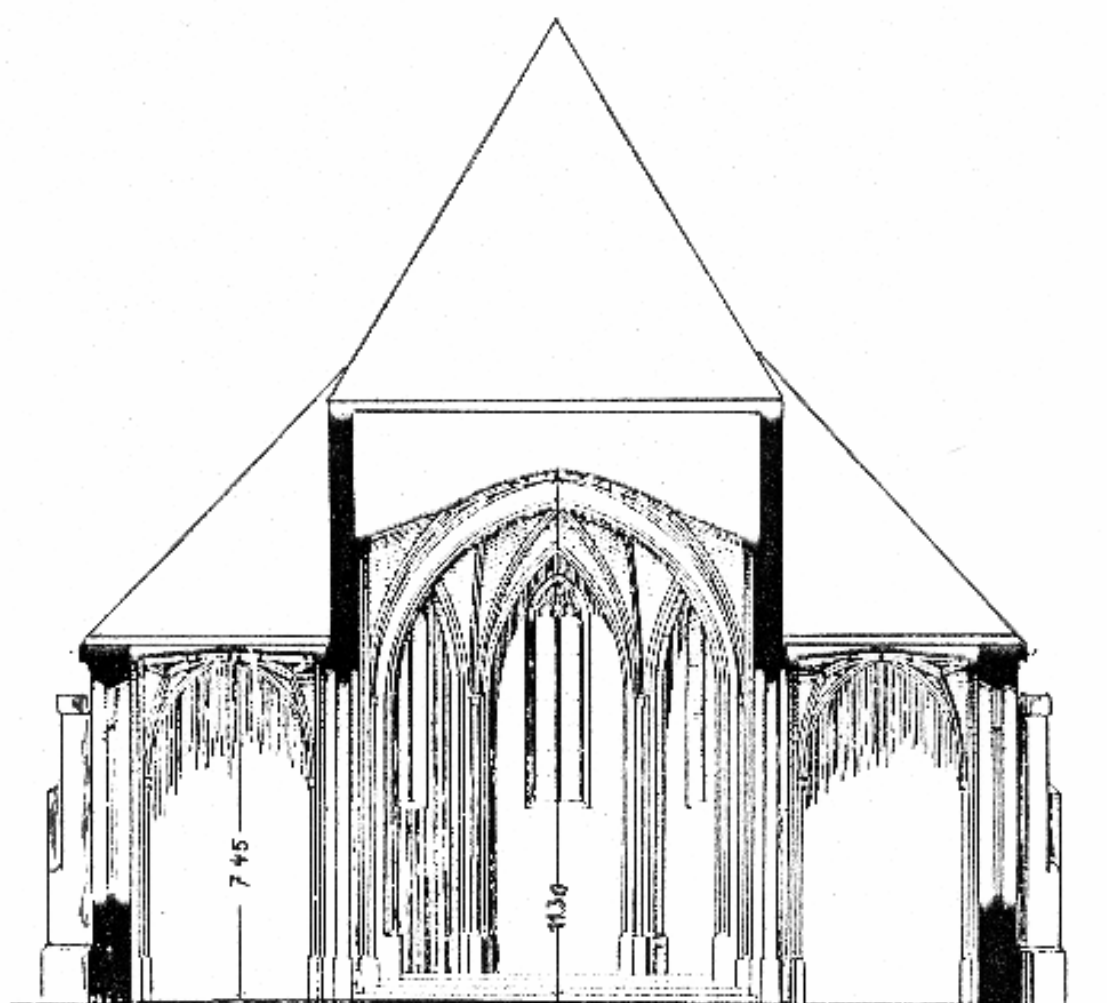
QUERSCHNITT
