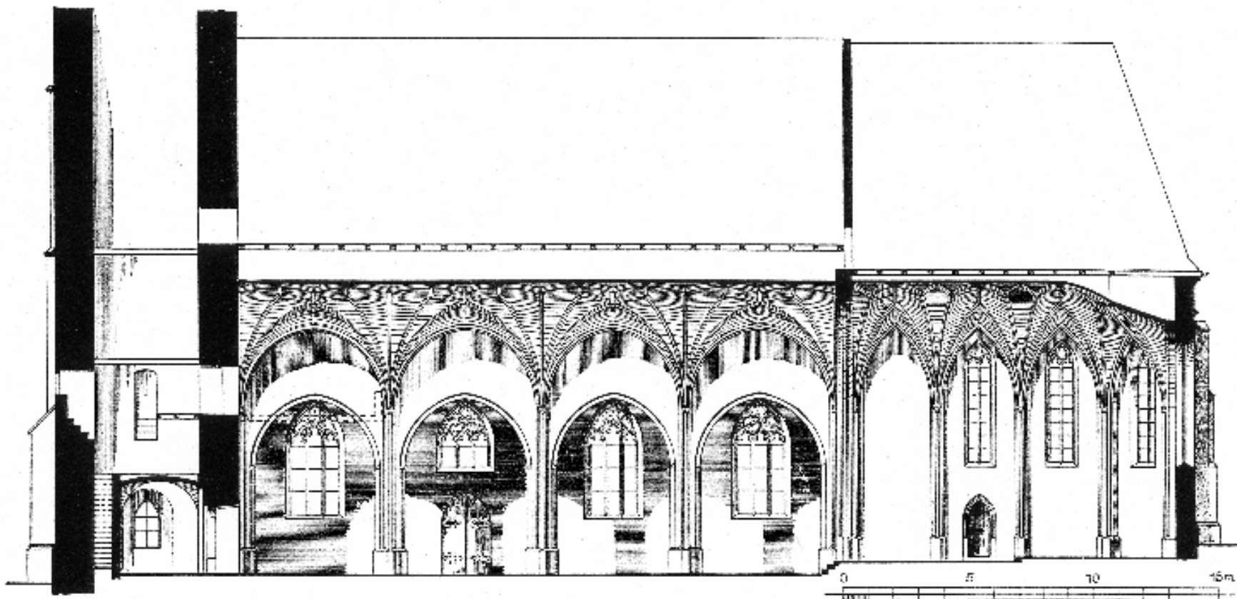
LÄNGSSCHNITT
