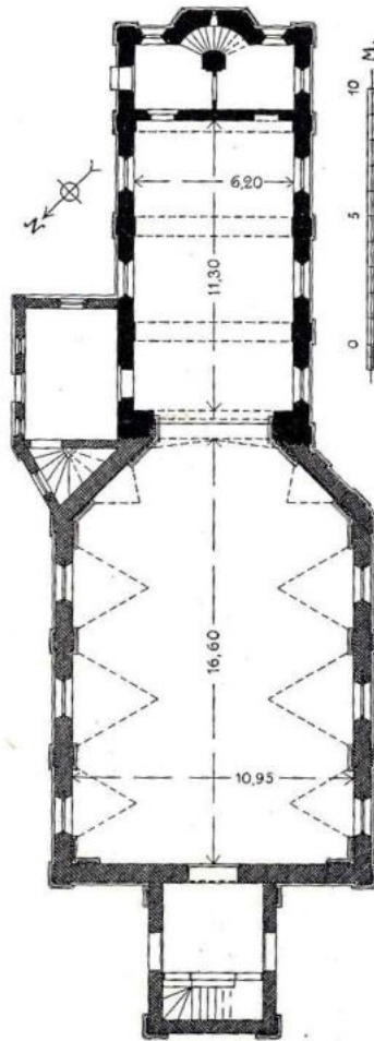
Fig. 34. Dreifaltigkeit. Kirche. Grundriß.
