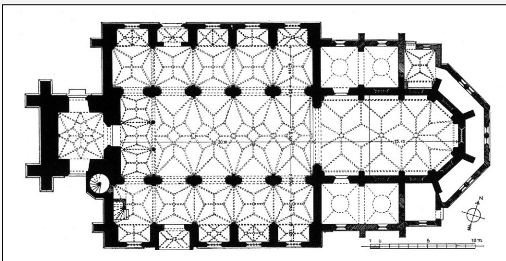
Grundriss der Stadtpfarrkirche Mariä Himmelfahrt Vilsbiburg mit der neun Rauten Hans Wechselberger Gewölbefiguration im Langhaus. In der Mitte des Langhauses das Heilig Geistloch.
